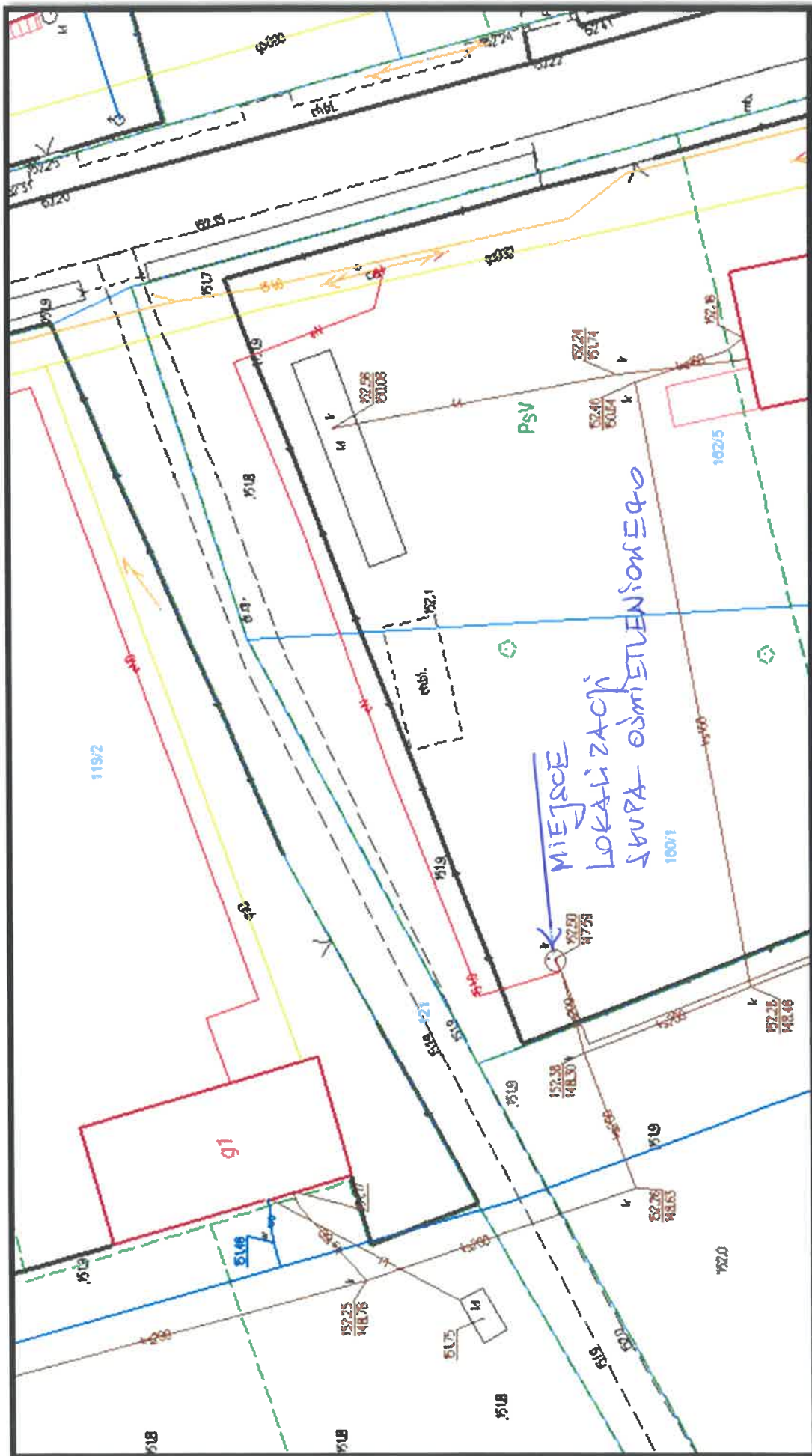
Szkic sytuacyjny budowy oświetlenia ulicznego w Ślężakach na działce nr ewid. 160/1
